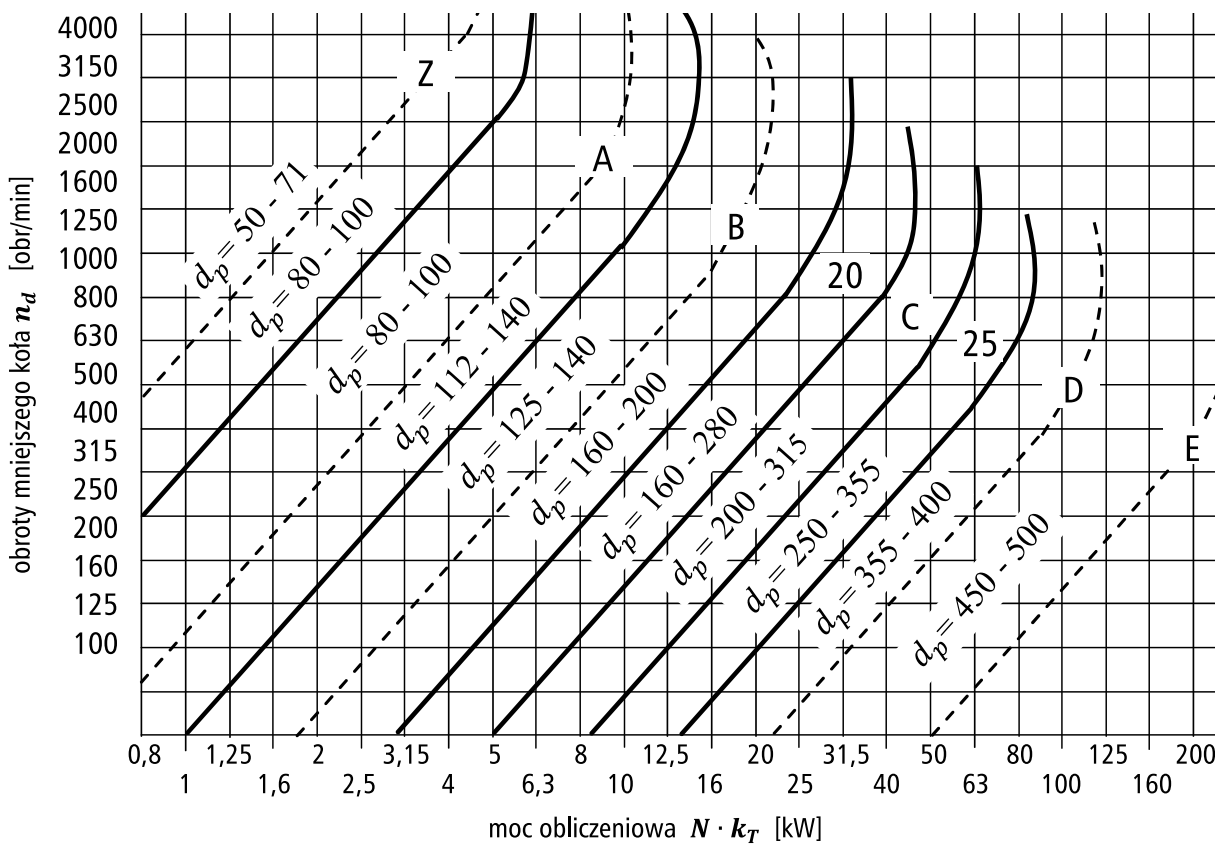
Rys. 3.1. Wykres wstępnego doboru wielkości przekroju pasa normalnoprofilowego
